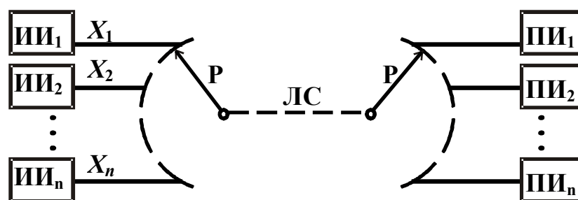
Рис. 1.7. Многоканальная система с временным разделением
