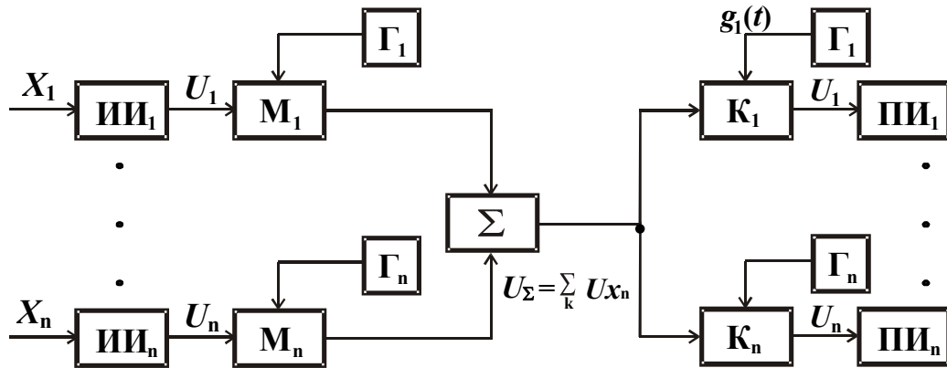
Рис. 1.13. Многоканальная система с корреляционным разделением
