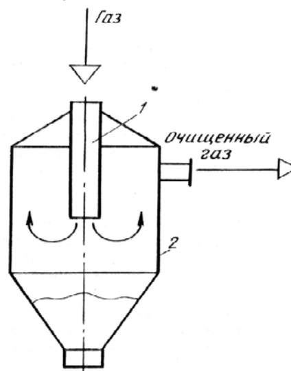
Рис.7.7. Радиальный пылеуловитель 1-входной патрубком; 2- корпус.
