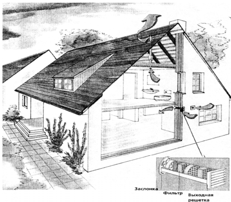
Рис. 8.7. Устройство вентиляционного канала
