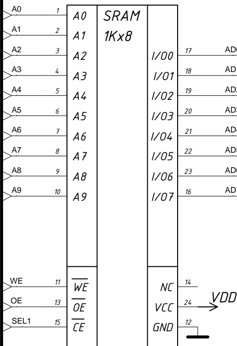
DD6 6108
