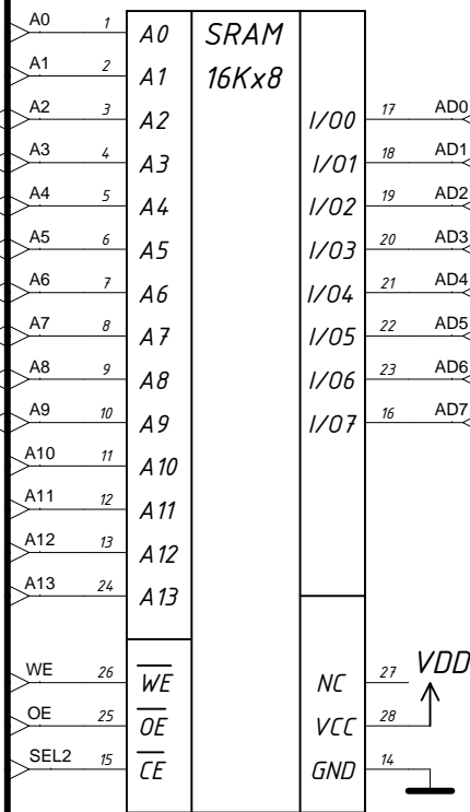
DD8 CY62128
