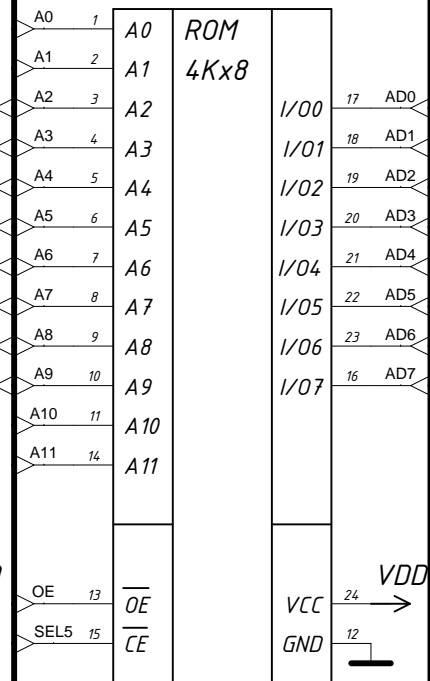
DD10 2732
