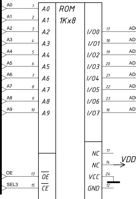
DD7 2708
