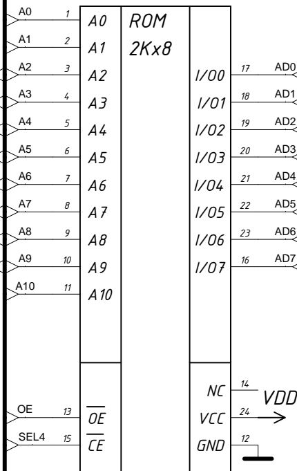
DD9 2716
